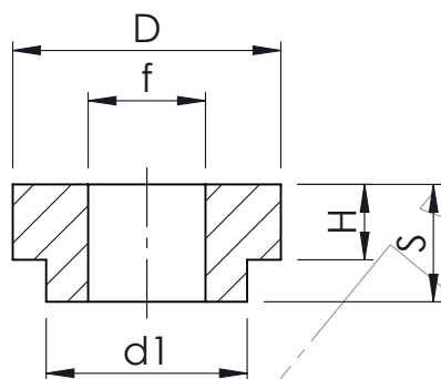
SEZIONE B-B
