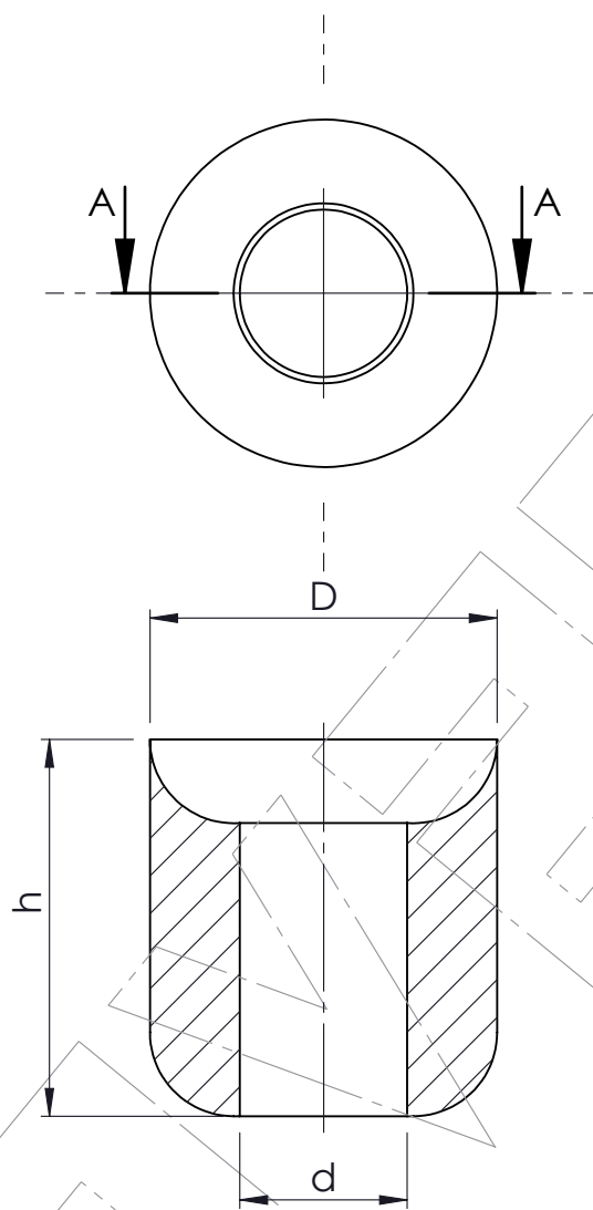
SEZIONE A-A
