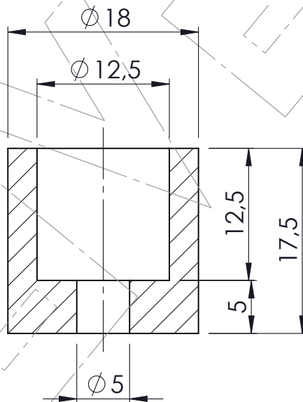
SEZIONE A-A
