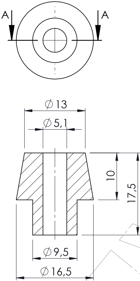
SEZIONE A-A
